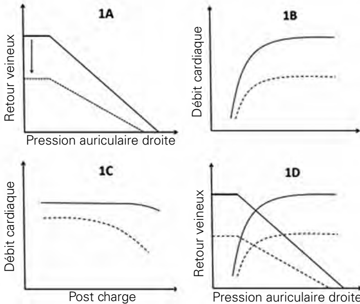
Figure 1 : Courbes de retour veineux : une hypovolémie entraîne une baisse du retour veineux (flèche) et une augmentation de la résistance au retour veineux (diminution de la pente) (Figure 1A). Courbes de fonction ventriculaire gauche normale (trait plein) et altérée (trait pointillé) selon la précharge. La partie pentue initiale des deux courbes traduit un état de précharge dépendance (Figure 1B). Courbes de fonction ventriculaire gauche normale (trait plein) et altérée (trait pointillé) selon la postcharge (figure 1C). Le croisement des courbes de la Figure 1A et 1B correspond à une mesure instantanée de débit cardiaque pour un patient donné (Figure 1D).
